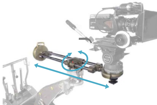
GF-Mini Bangi mit Standard 75cm Rohre auf Dolly
