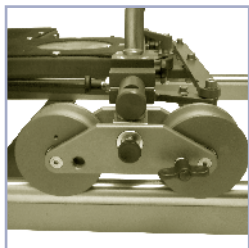
Schienenradsatz
