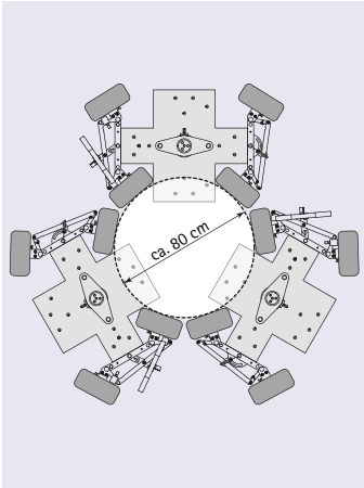
Extrem enge Kreisfahrten
